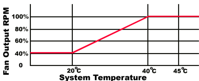
Fan Output Chart
